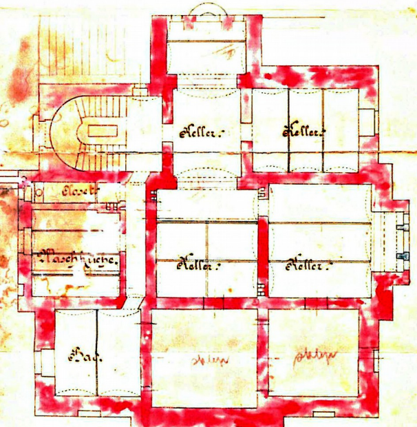
Plan vom Souterrain.
