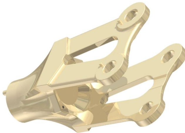
Obr. 1: závěs listu
