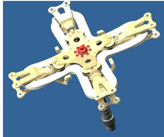
Obr. 3: rotorová hlava
