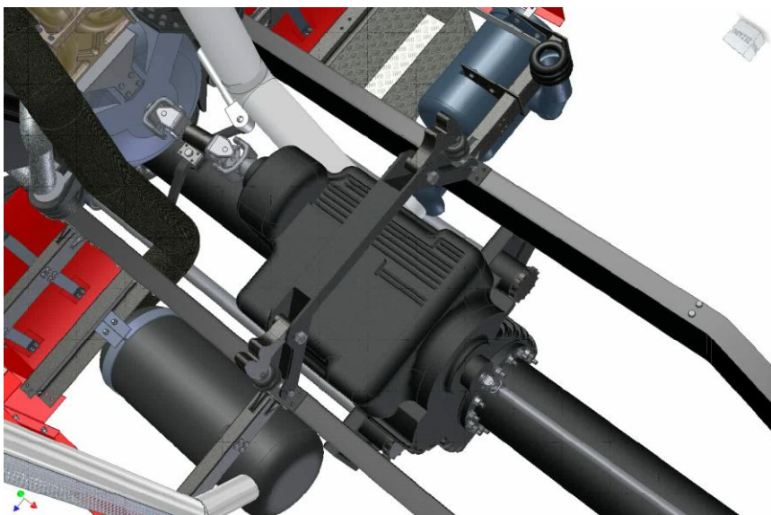
Obr. 2: převodový agregát
