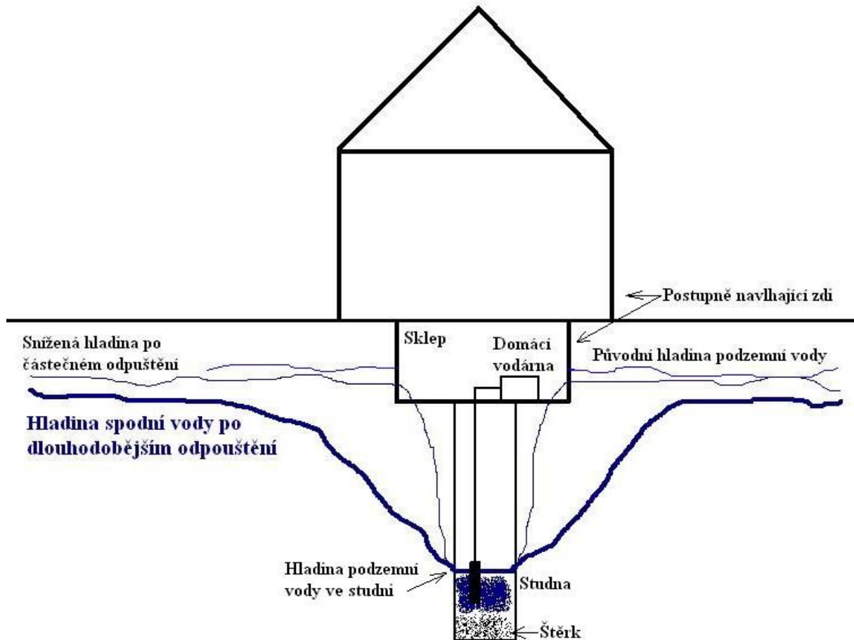
Obr. 1 Snižování hladiny spodní vody
