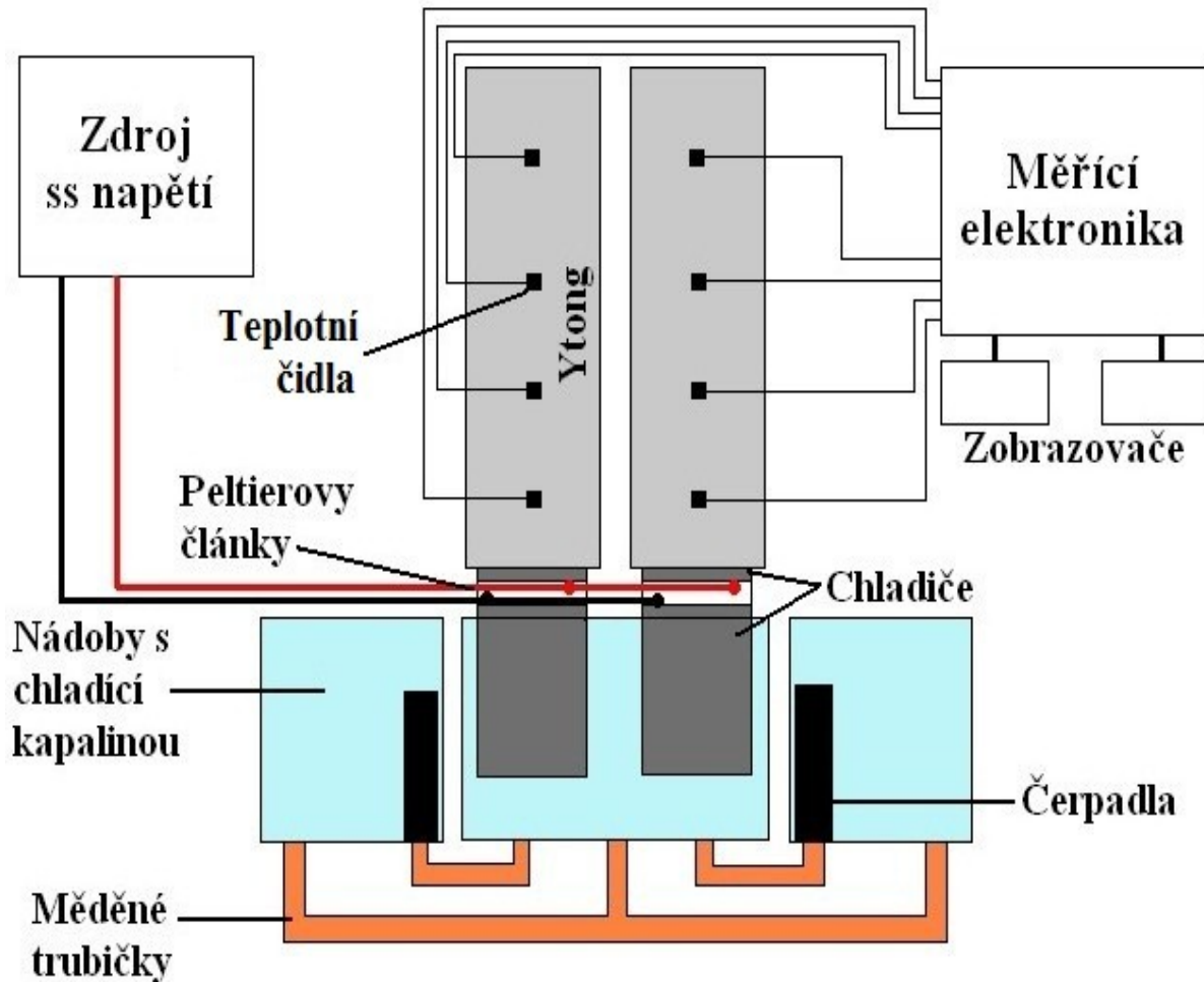
Obr. 2 Schéma demonstrační aparatury pro měření prostupu tepla suchým a mokrým zdivem
