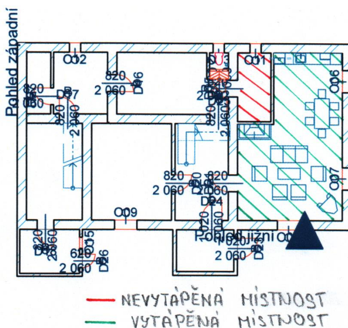
Obrázek č. 9 – půdorys rekreačního objektu [9]
