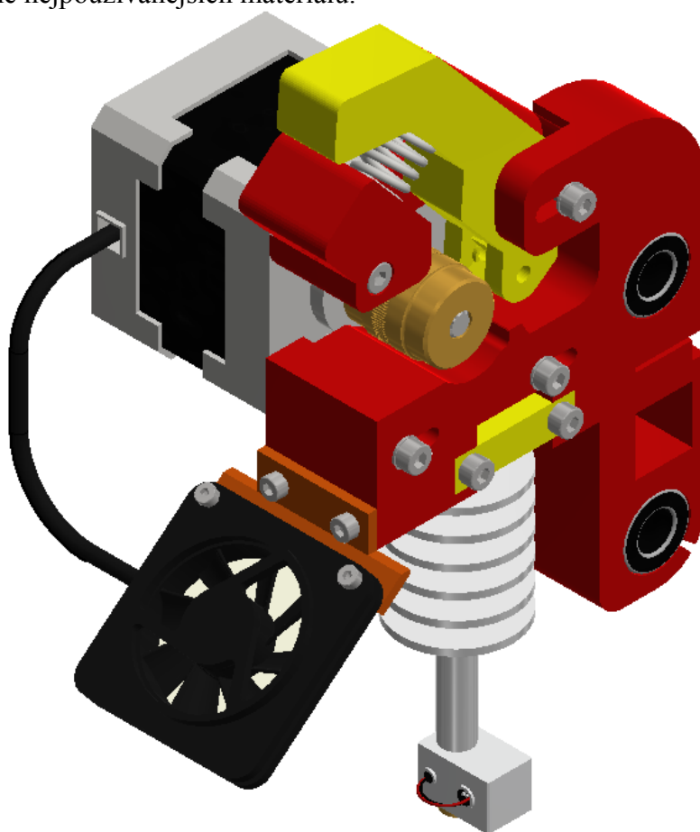
Obr. 1: tisková hlava (extruder)
