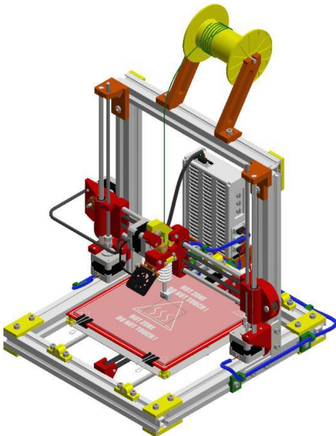
Obr. 2: celkový pohled
