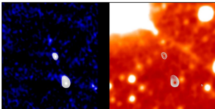
Obrázek 6 – proud částic směřující do středu černé díry, snímek ARG000345v (zdroj: zooniverse.org)
