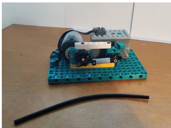
Obrázek 7 : Kompresor pro tlakový vzduch z dílů stavebnice Lego Technic
