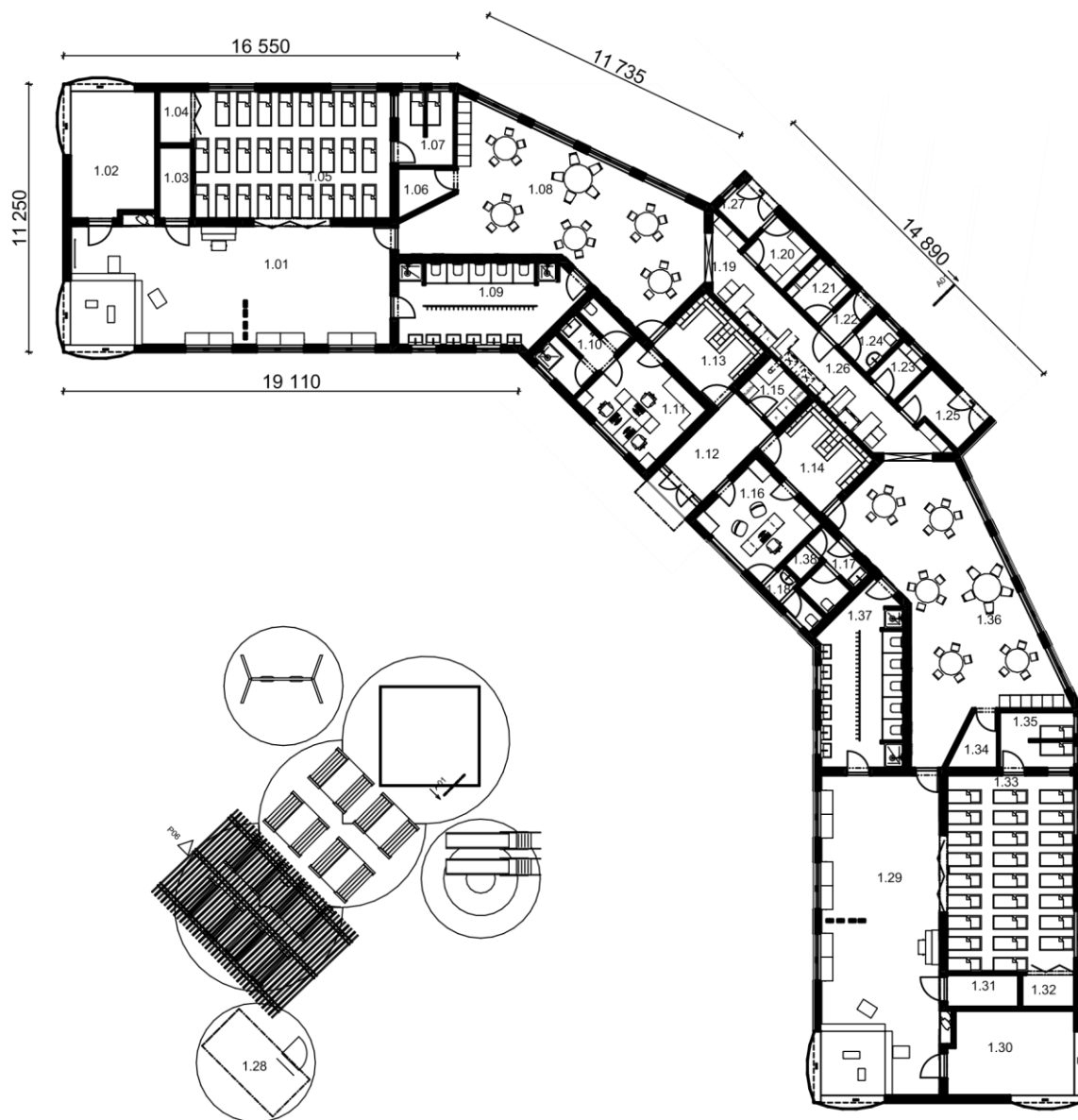
Obr. 2 : Půdorys školky
